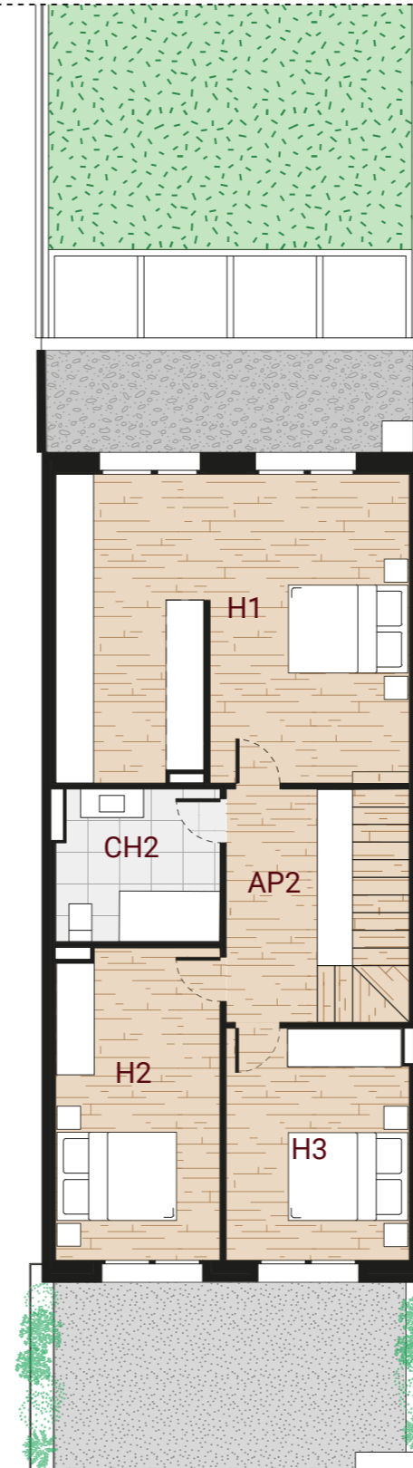
Planta 1
