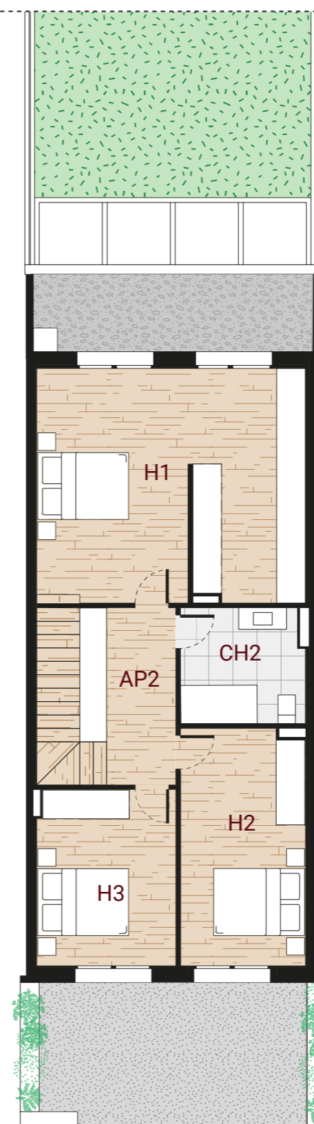
Planta 1
